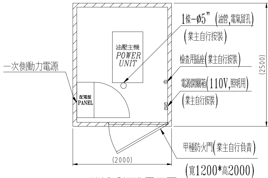
機械房標準平面圖
